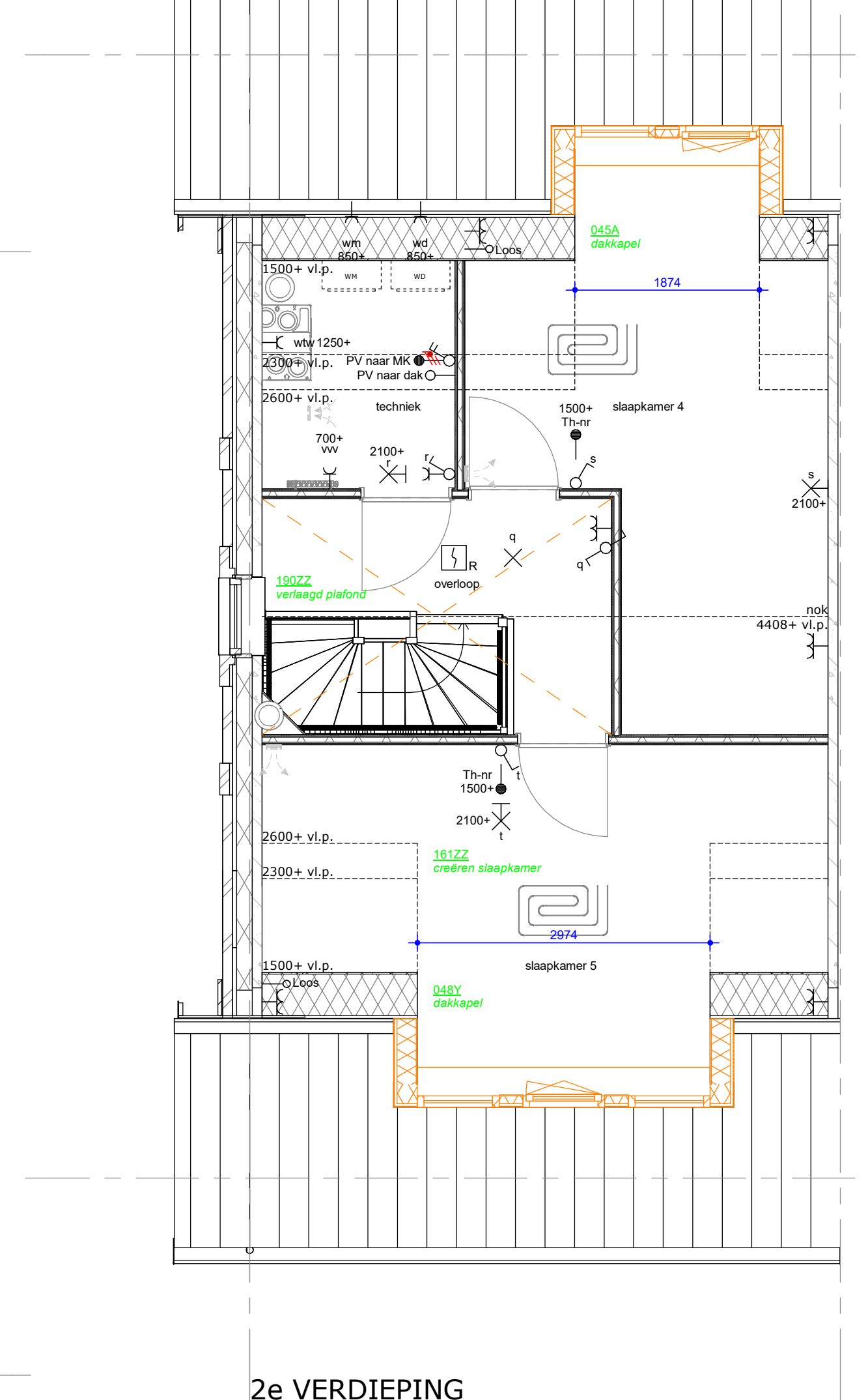
2e VERDIEPING
