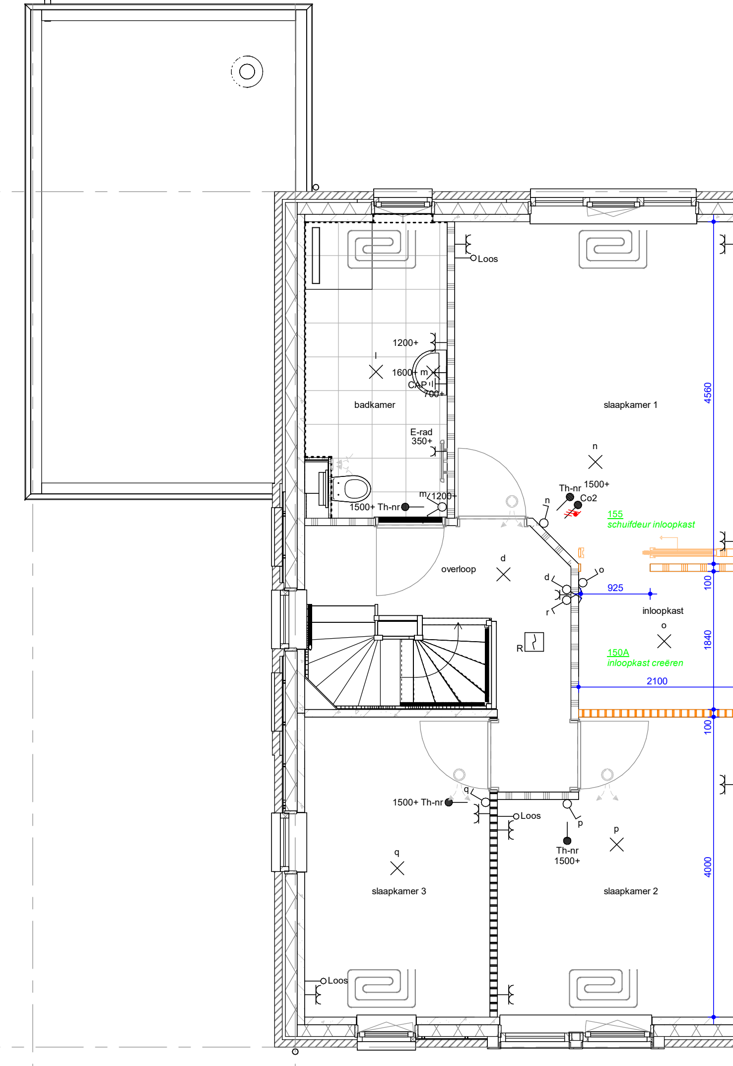
1e VERDIEPING
