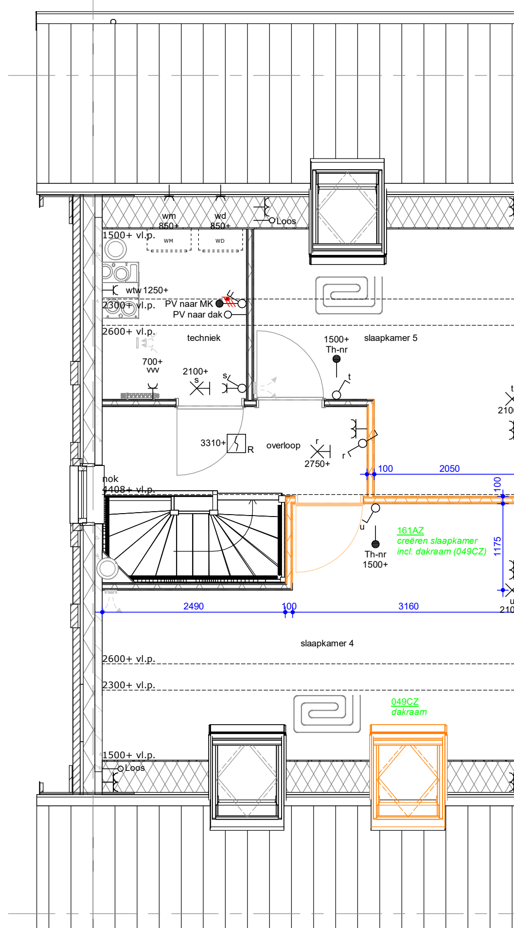
2e VERDIEPING
