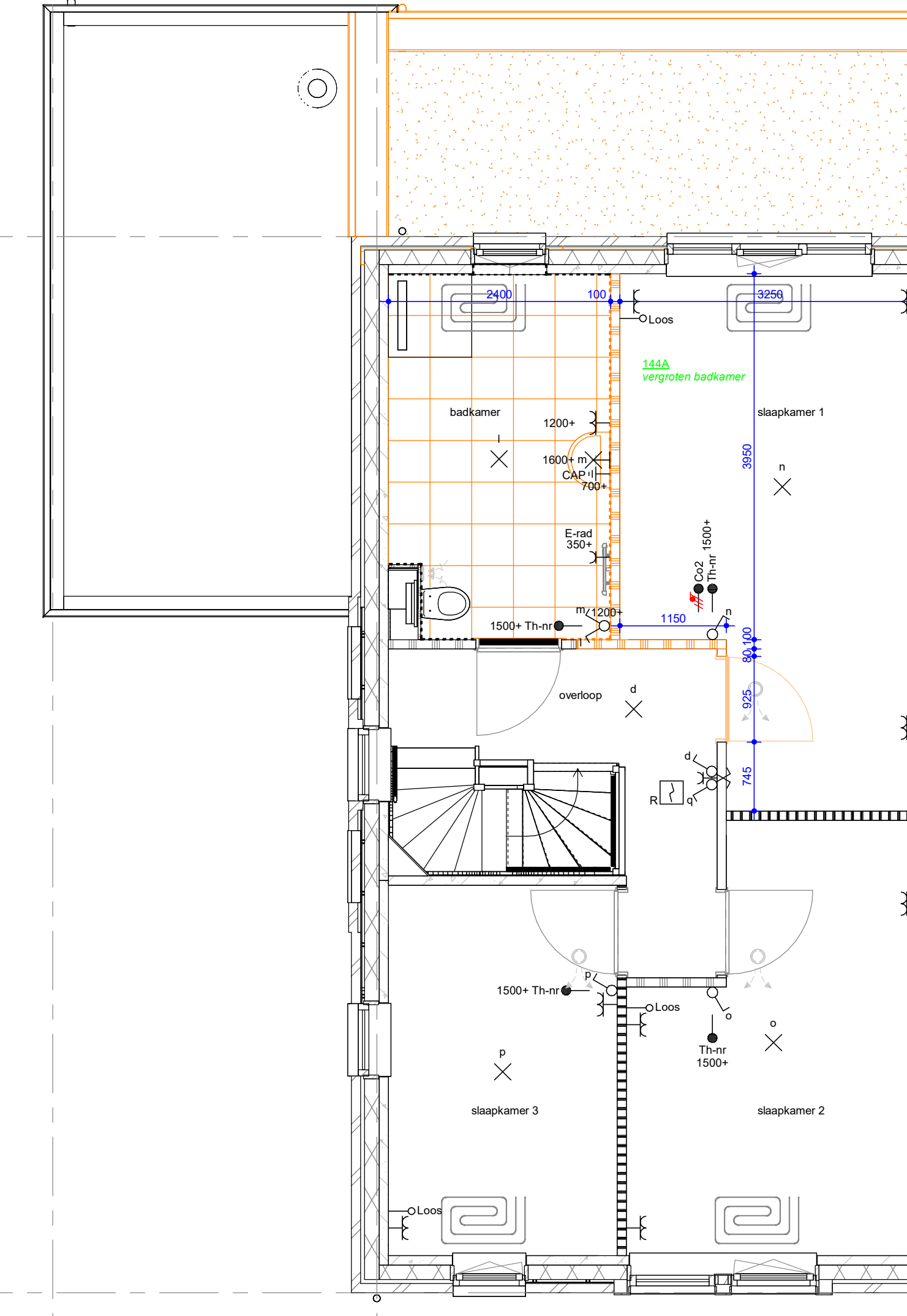
1e VERDIEPING
